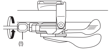
VİTES KOLU AYAR VIDASI
