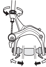
FREN BACAĞI AYAR NOKTASI
